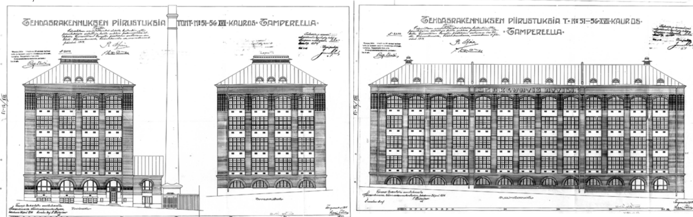
Attilan julkisivupiirroksiset länteen, itään ja pohjoiseen. (Heikki Tiitola 1914, Tampereen rakennusvalvonna arkisto)
